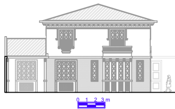
Elevation 02
