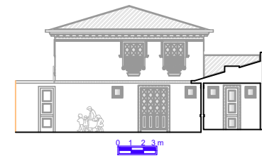
Elevation 04
